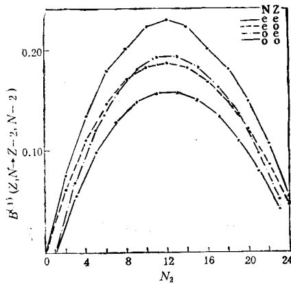
图1 约化 \alpha 转移率 B^{(1)}(Z, N \rightarrow Z-2, N-2) 和 N_2 的关系
