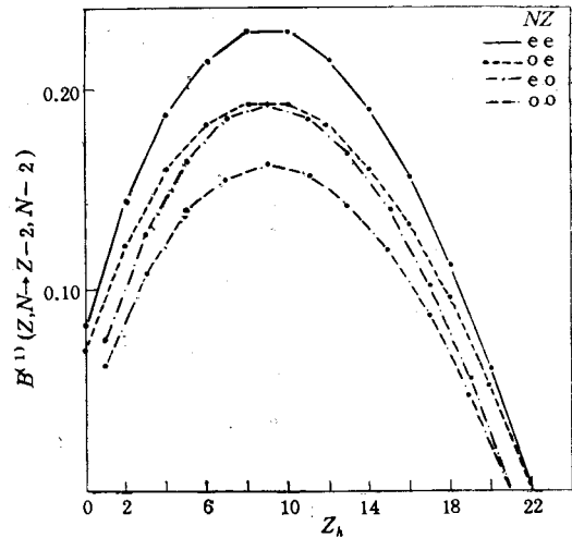
图2 约化 \alpha 转移率和 Z_h 的关系 B^{(1)}(ZN \rightarrow Z-2, N-2)
